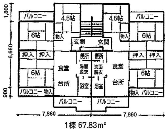
<間取り図(1)>
