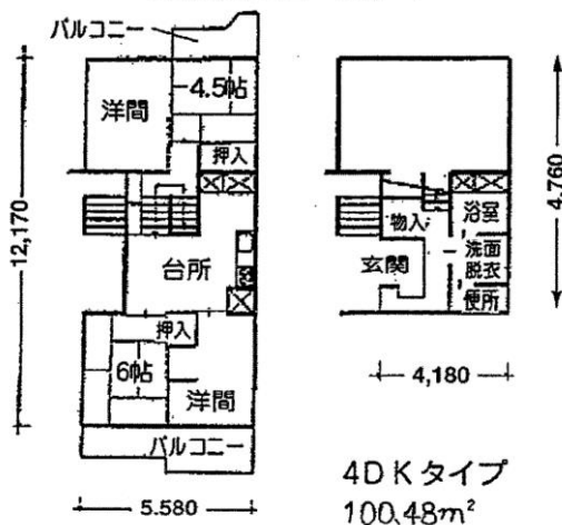
<間取り図 (3)>
