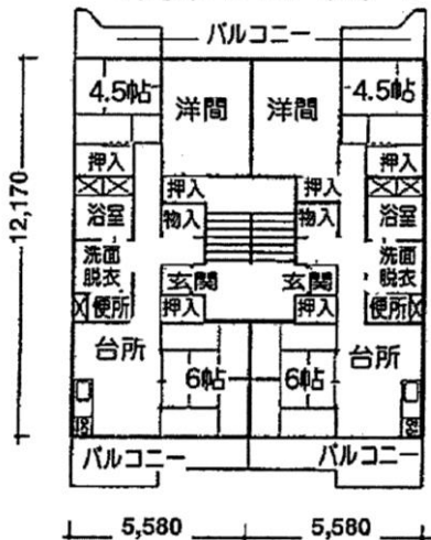
<間取り図 (2)>
