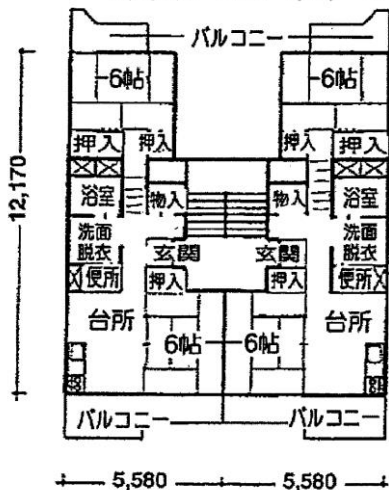
<間取り図 (1)>
