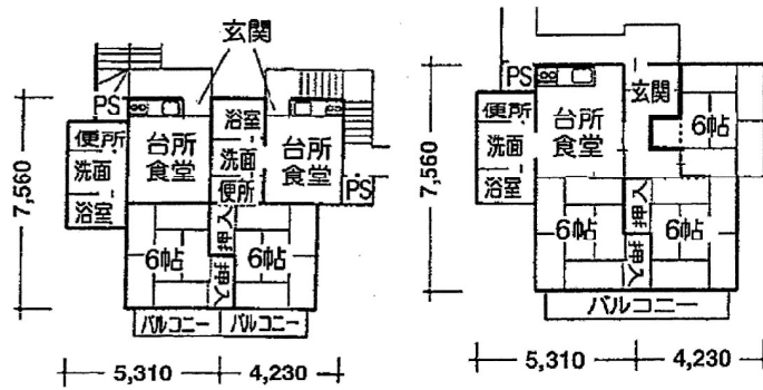
3棟Aタイプ 32.59m 2 3棟Bタイプ 32.59m 2 3棟Cタイプ 77.31m 2
