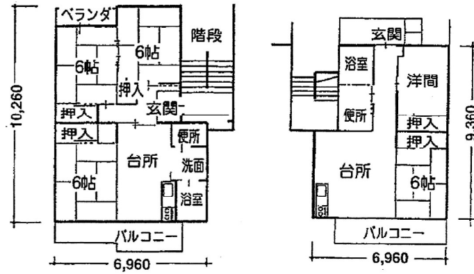
2棟Aタイプ 71.15m 2 2棟身障者向住宅 68.23m 2
